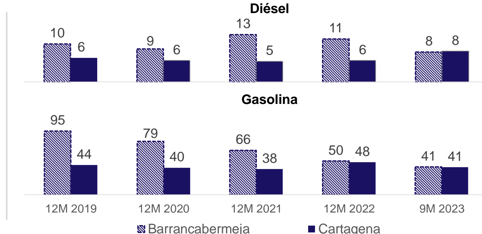
Cantidad Azufre en Diesel y Gasolina (ppm)** 2019 - 9M 2023
